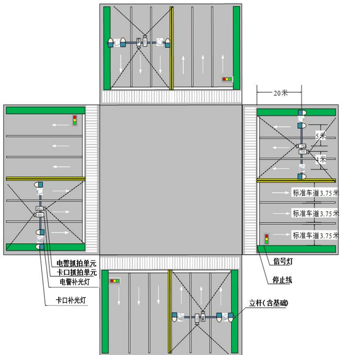
路口电警卡口部署示意图
