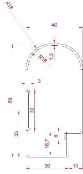
(床横梁效果示意图)
