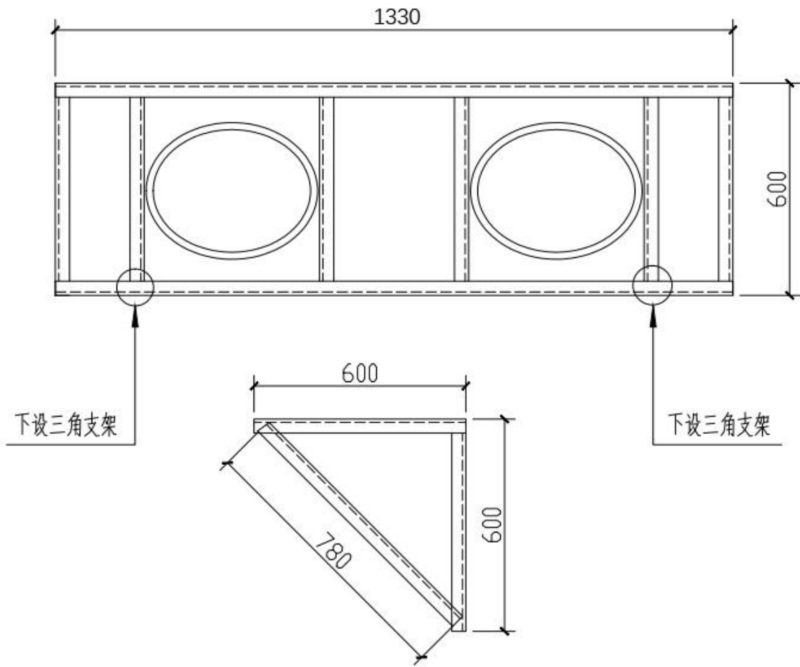
宿舍盆架做法示意图 1:100
