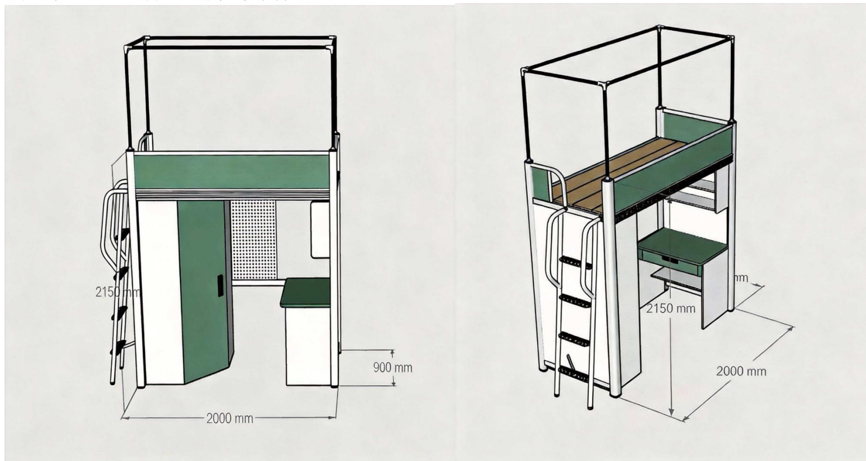
附：单人位侧入式公寓组合床参考结构图
