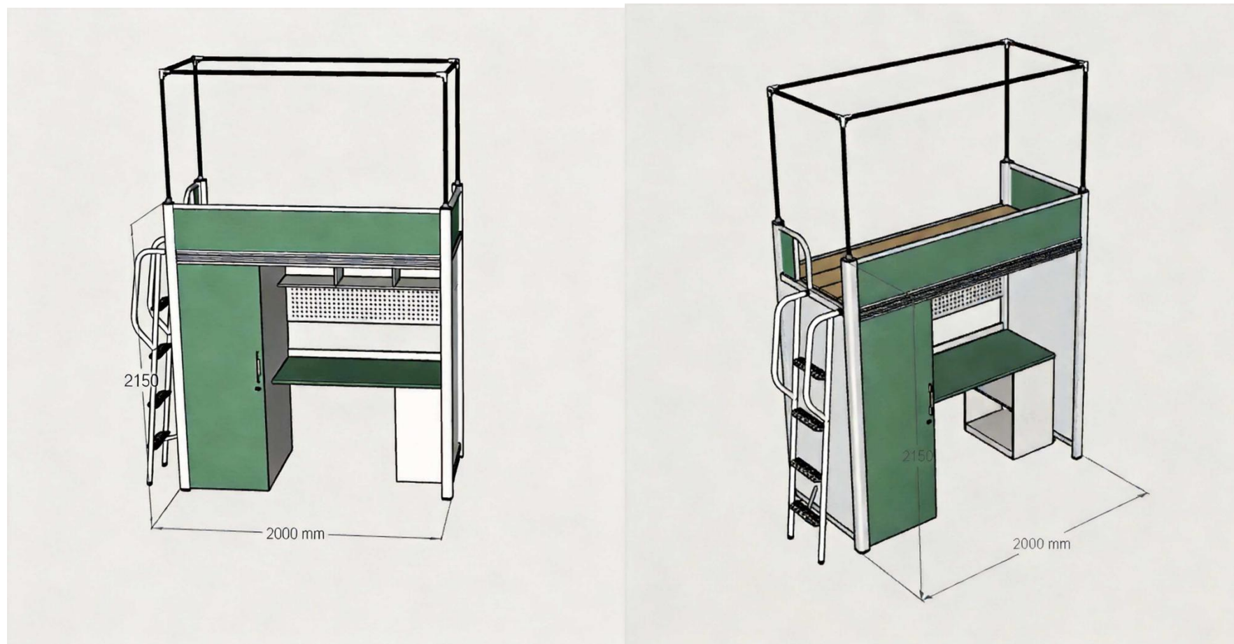
附：单人位侧爬梯公寓组合床参考结构图
