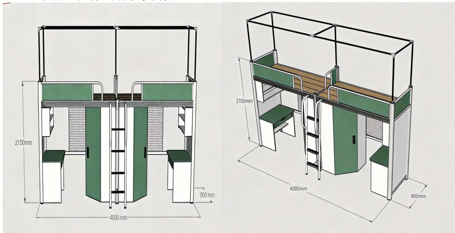
附：二人位侧入式公寓组合床参考结构图
