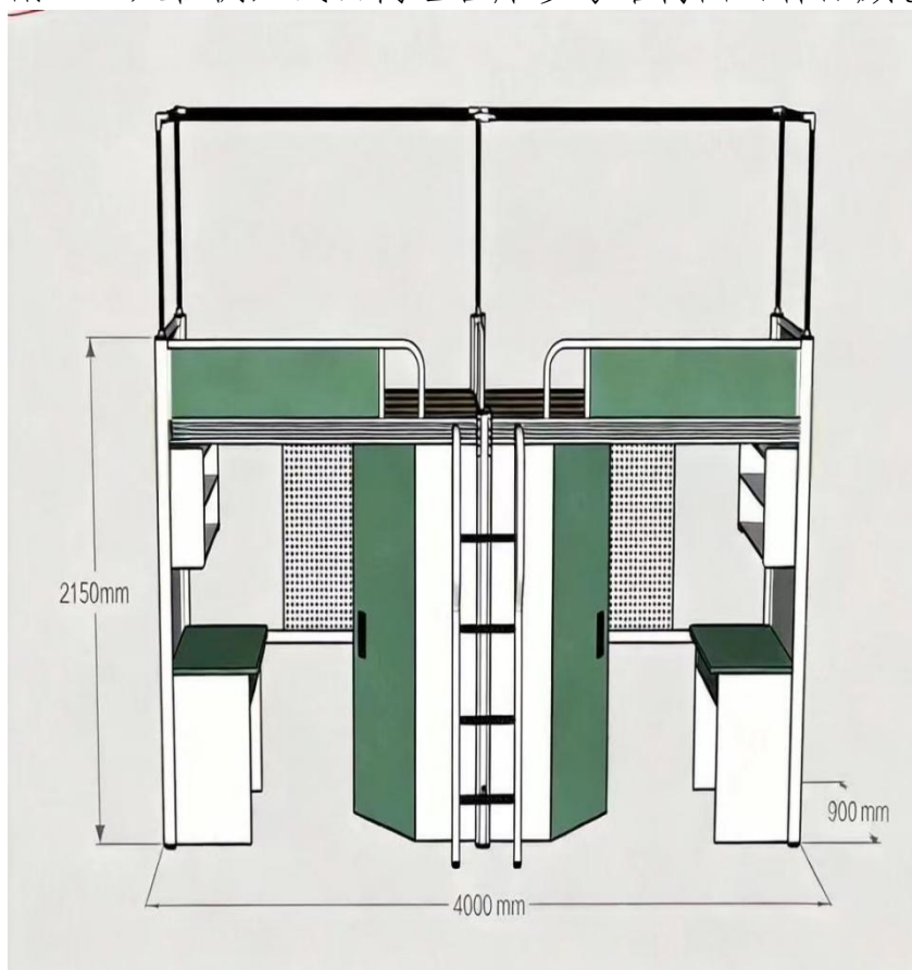
附：二人位侧入式公寓组合床参考结构图（样品颜色可自行选择）
