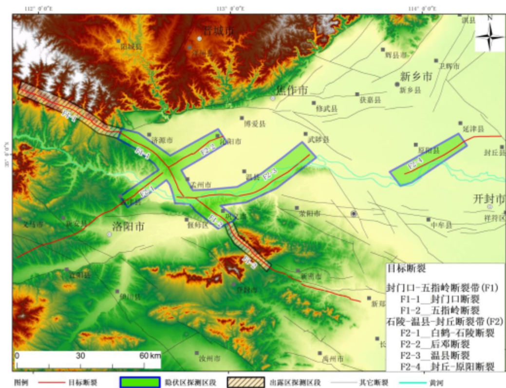
图 1 目标断裂与勘探区段分布示意图
