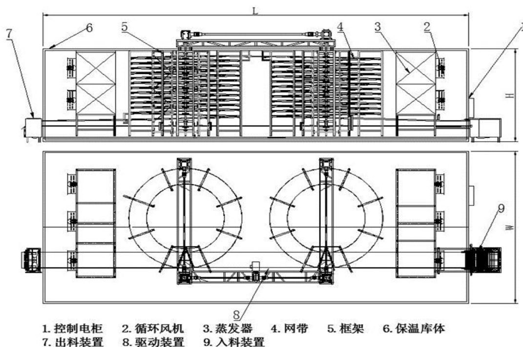
附图 1:双螺旋制冷机结构示意图，不作为实际用图
