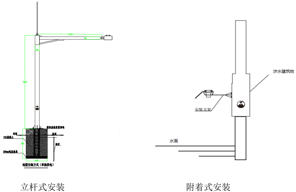
简易水位站安装示意图
