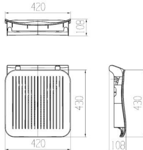
(坐板示意图)
