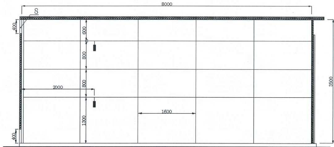
图 5—1 装烟室剖面结构示意图（气流下降式）
