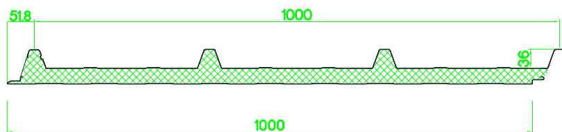
图 5 屋顶板视图
