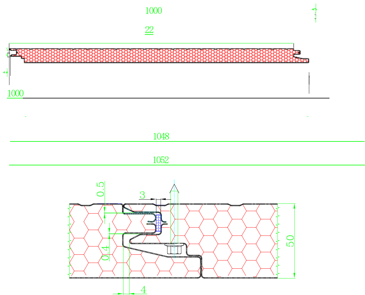
图4 墙板及连接图
