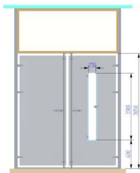
图 8 装烟室大门
