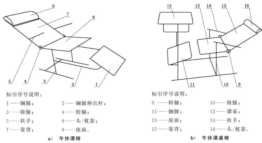
图 1 午休课桌椅典型结构示意图
