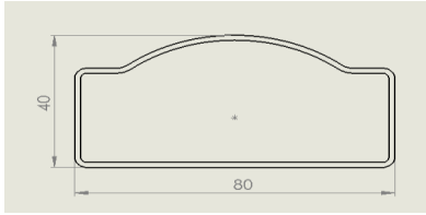
长横梁参考示意图
