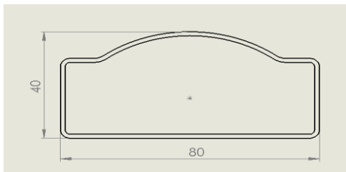
长横梁参考示意图
