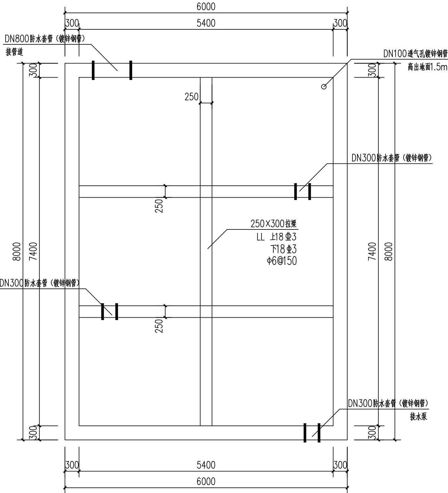
90m³三级沉淀池平面图
