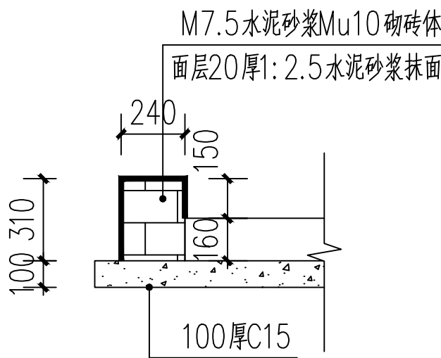
台阶2-2剖面图
