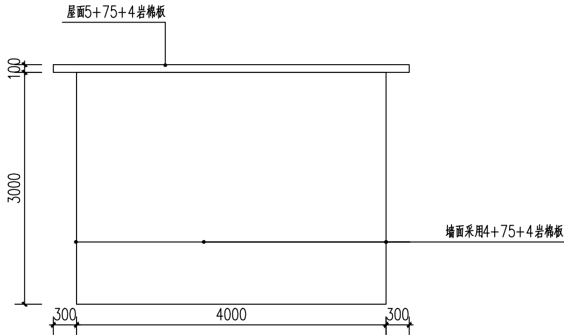
②—①轴立面图
