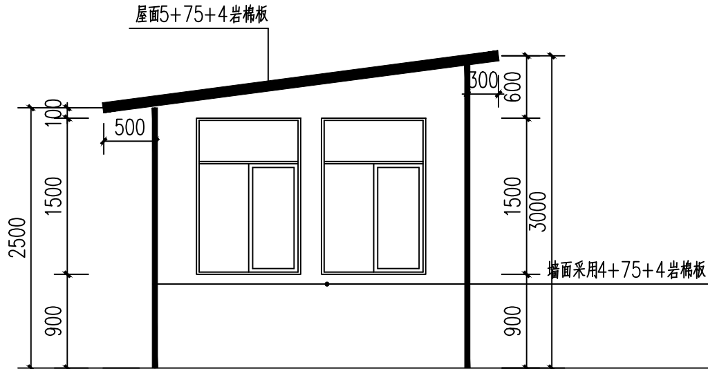
①—②轴立面图
