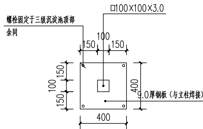
GZ 立柱基础图
