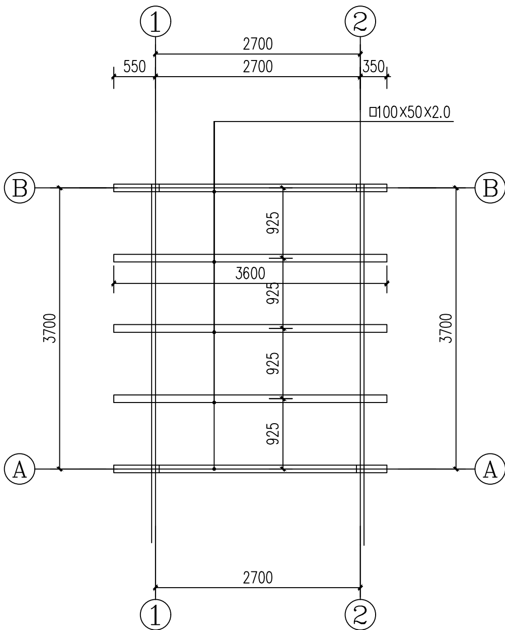
泵房屋面梁平面图
