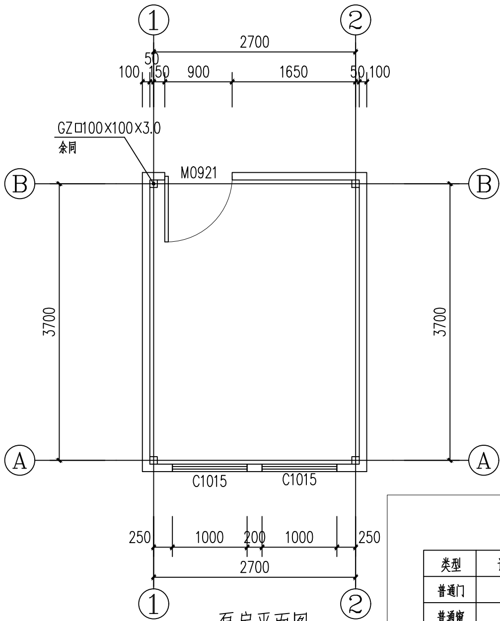
泵房平面图
