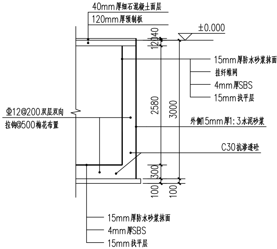
90m³三级沉淀池立面图
