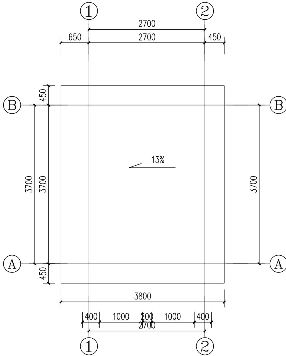
泵房屋面图
