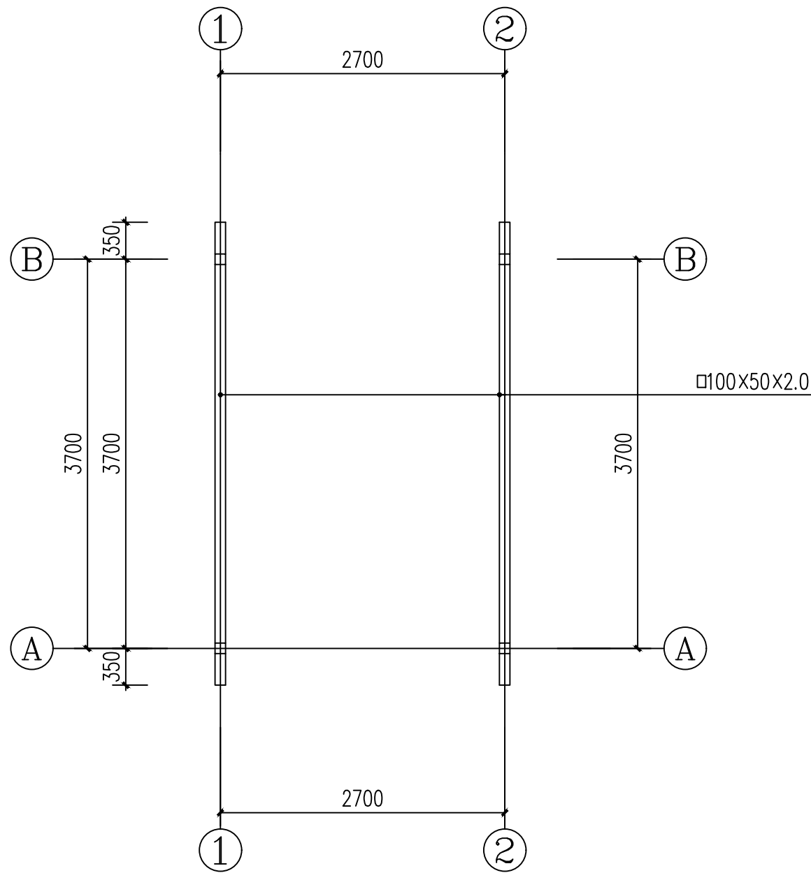
泵房屋面梁平面图
