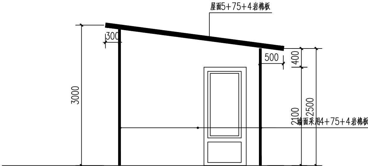
②—①轴立面图
