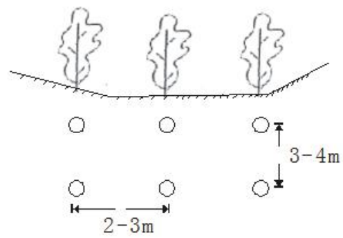
图2 造林图式
