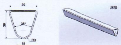
(床撑示意图)
