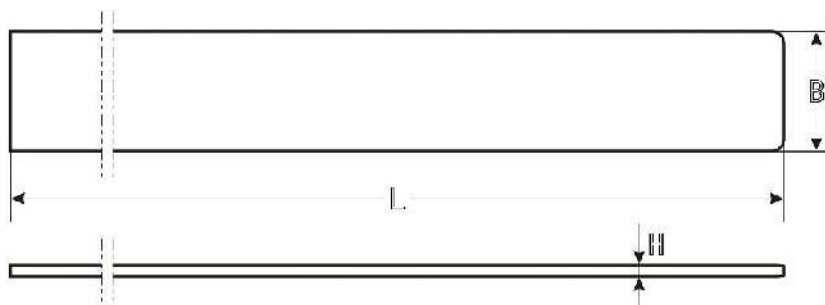
图 2 带体成品尺寸测量部位示意图
