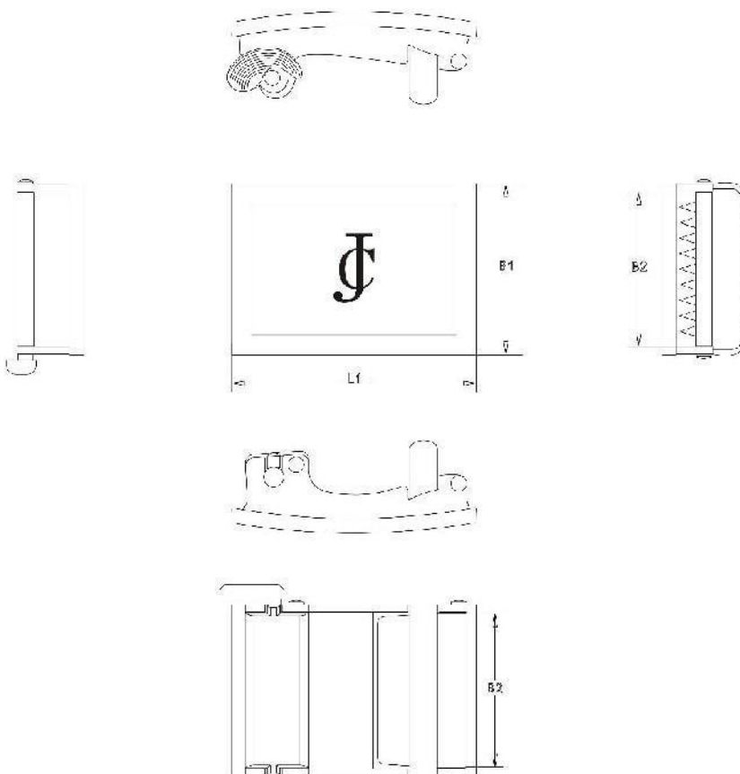
图 3 带体成品尺寸测量部位示意图
