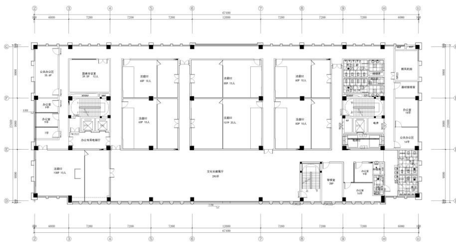
三层平面布置图 Scale: 1:100
