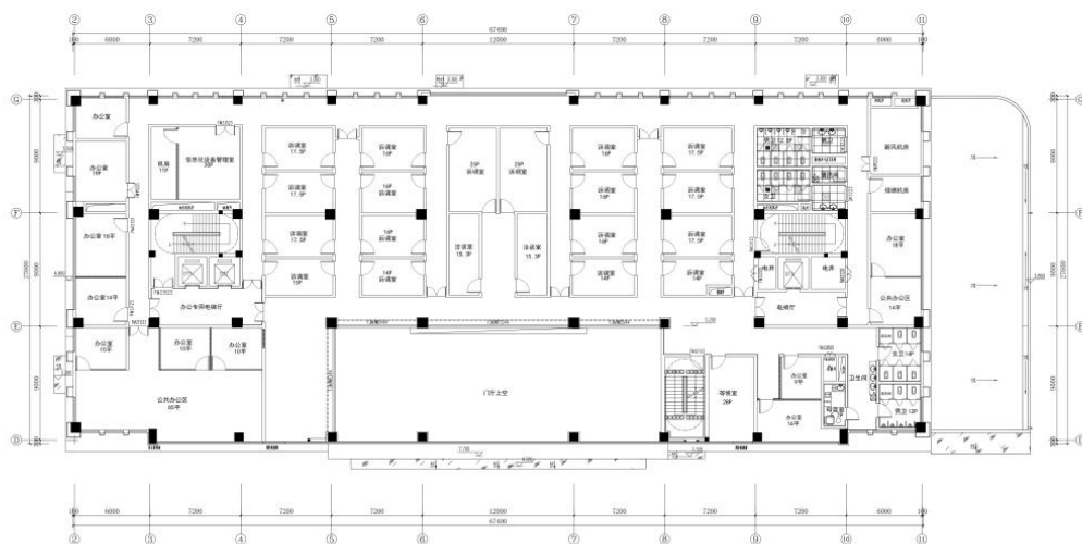
二层平面布置图 Scale: 1:100
