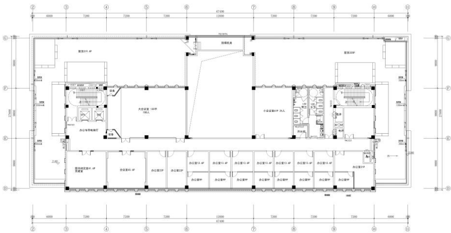
五楼平面布置图 Scale: 1:100
