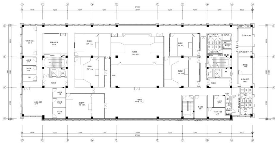
四楼平面布置图 Scale: 1:100
