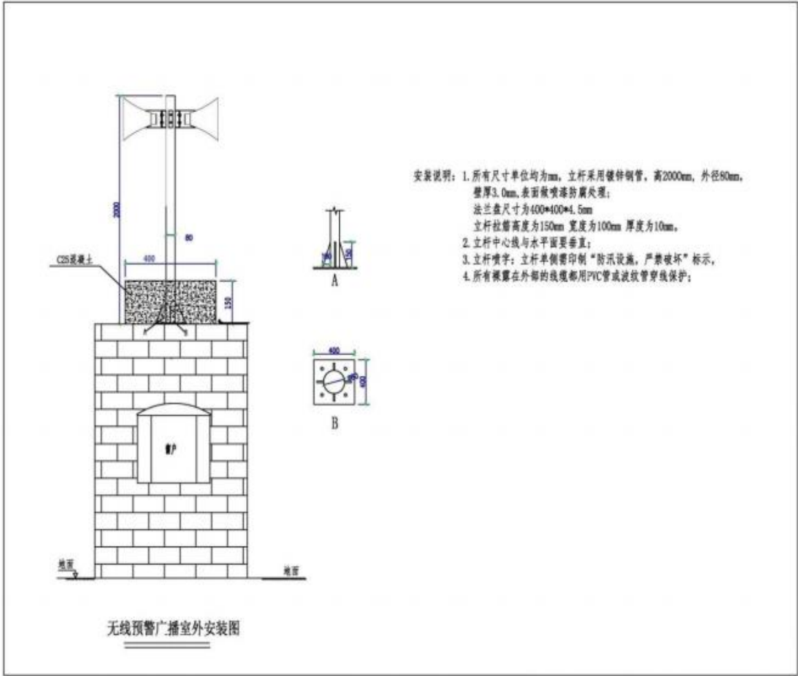
图 4.1-1 无线广播安装示意图
