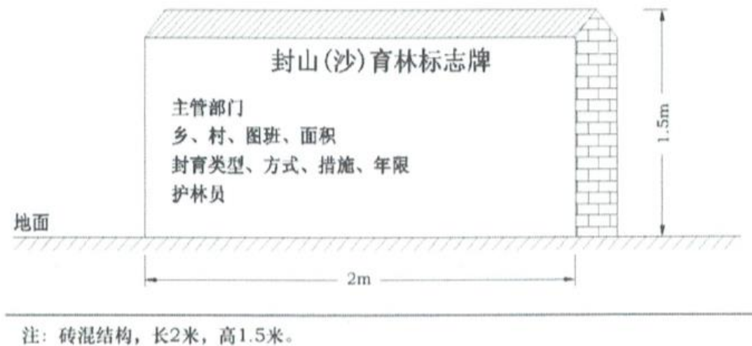
封山育林区标志牌示意图
