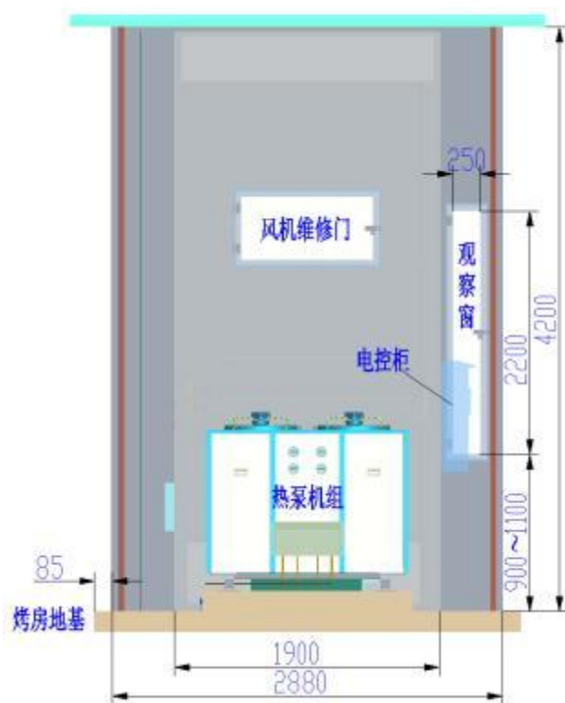
图 3 烤房正视图
