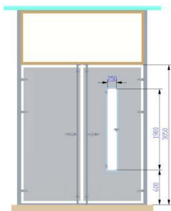
图 8 装烟室大门
