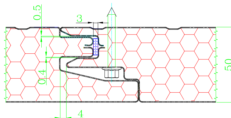
图4 墙板及连接图
