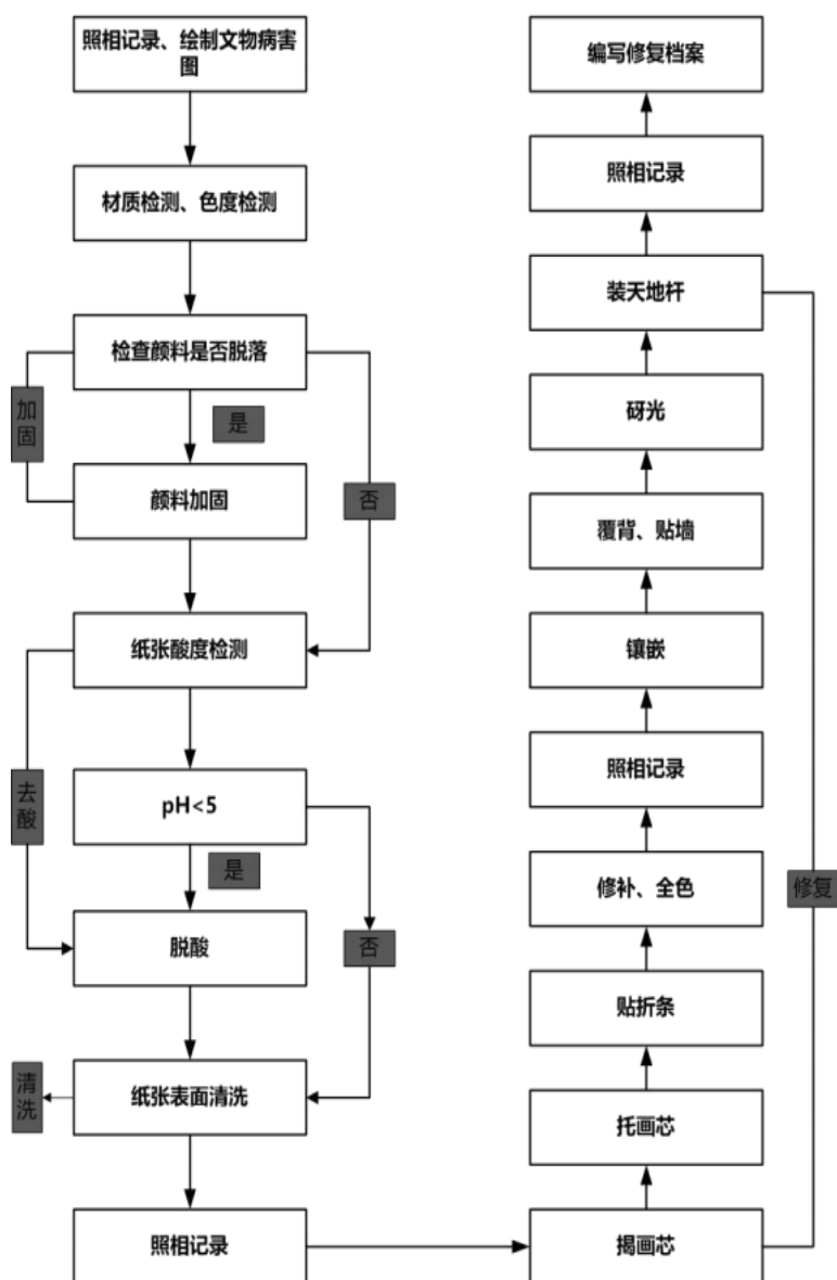
工艺流程图
