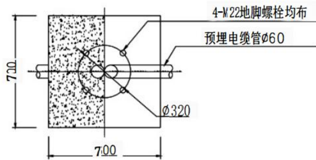
基础平面图
