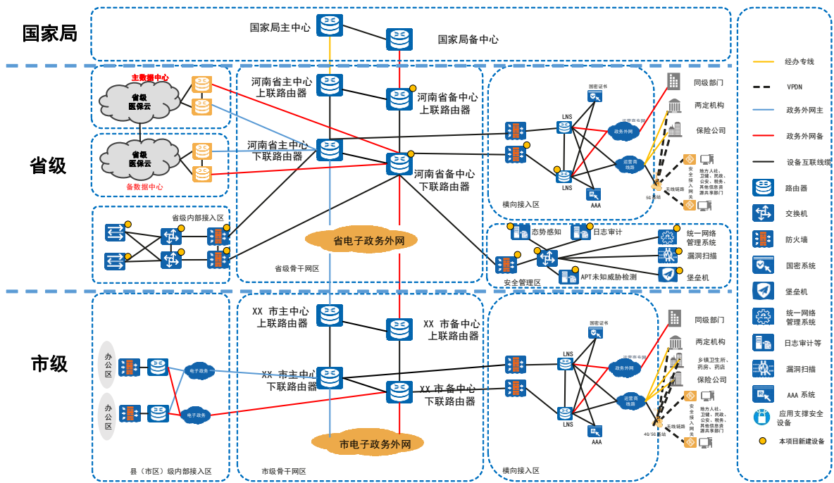
图 0-3 河南省医疗保障信息平台广域网网络架构图
